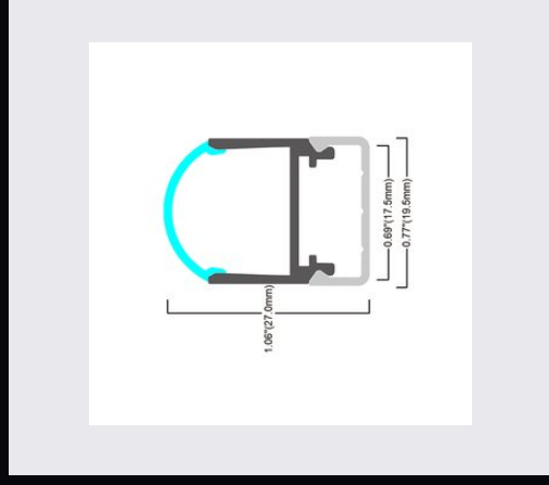
COUPE TECHNIQUE
